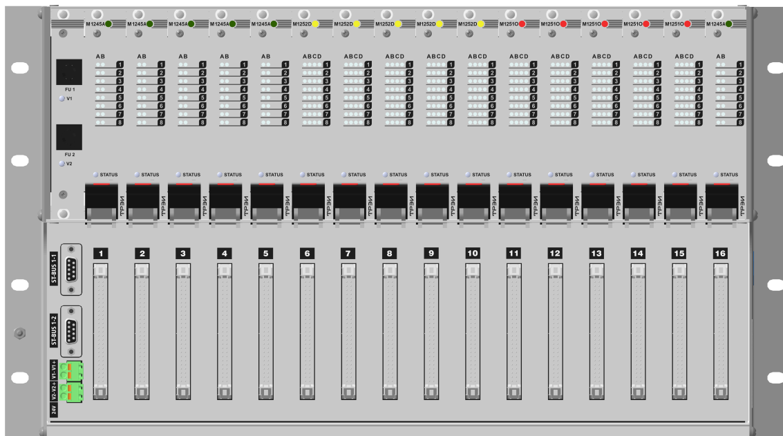
Рисунок 13 – Внешний вид передней панели каркаса CR6 IOR
