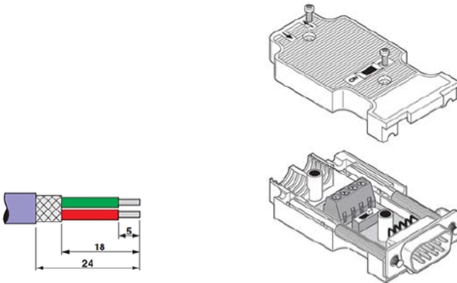
Рисунок 3 – Внешний вид соединителя CSB-1
