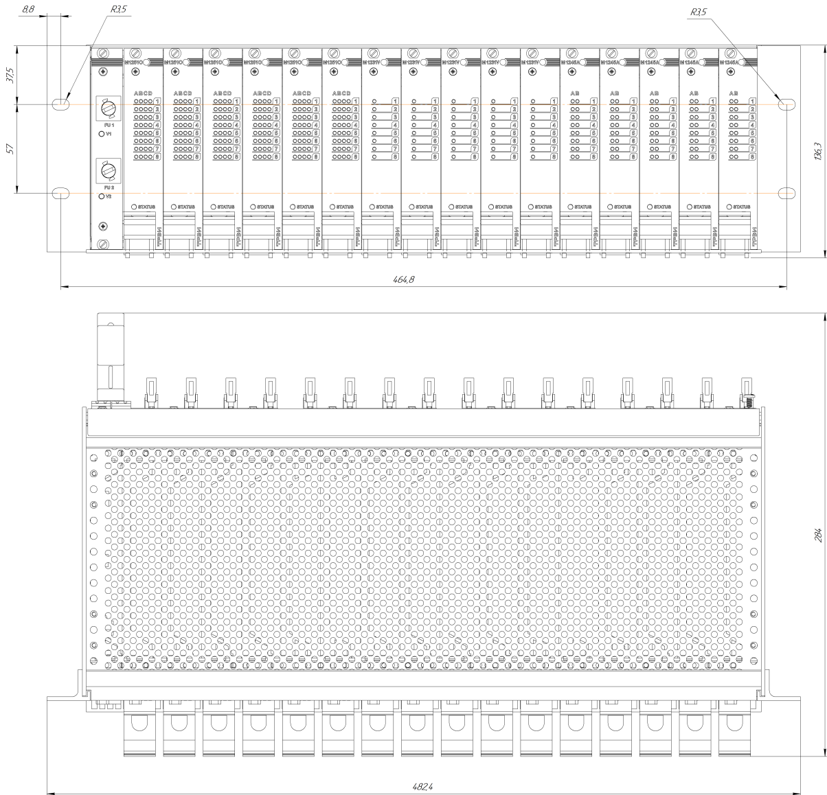
Рисунок 9 – Чертеж общего вида каркаса CR IOR с указанием габаритных размеров
