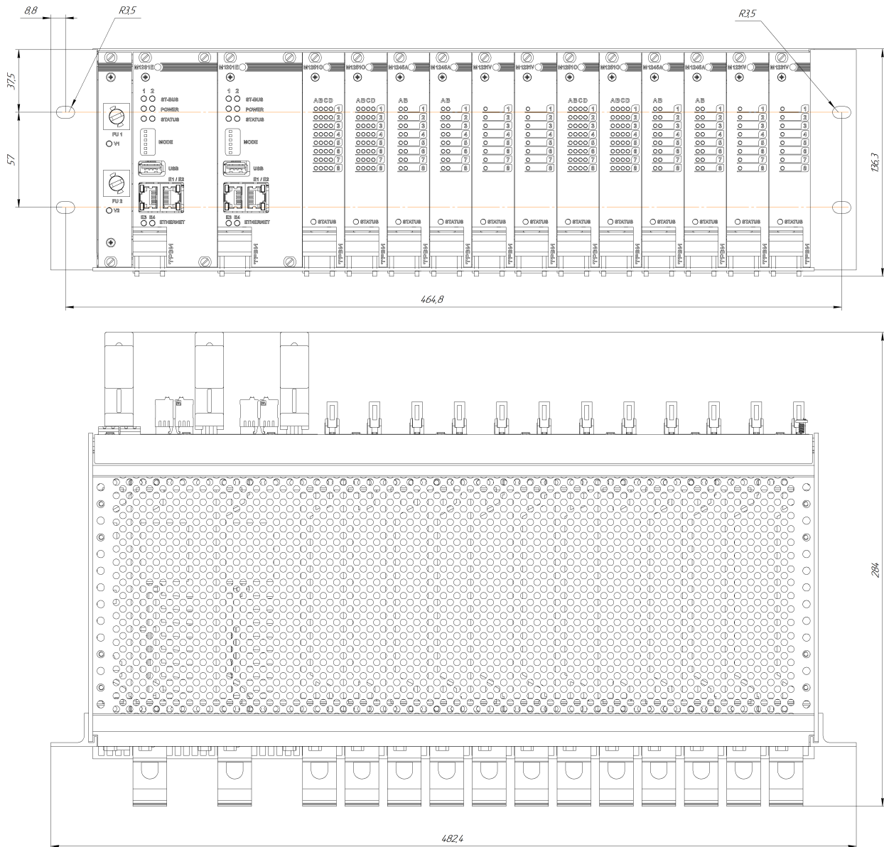
Рисунок 6 – Чертеж общего вида каркаса CR MR с указанием габаритных размеров
