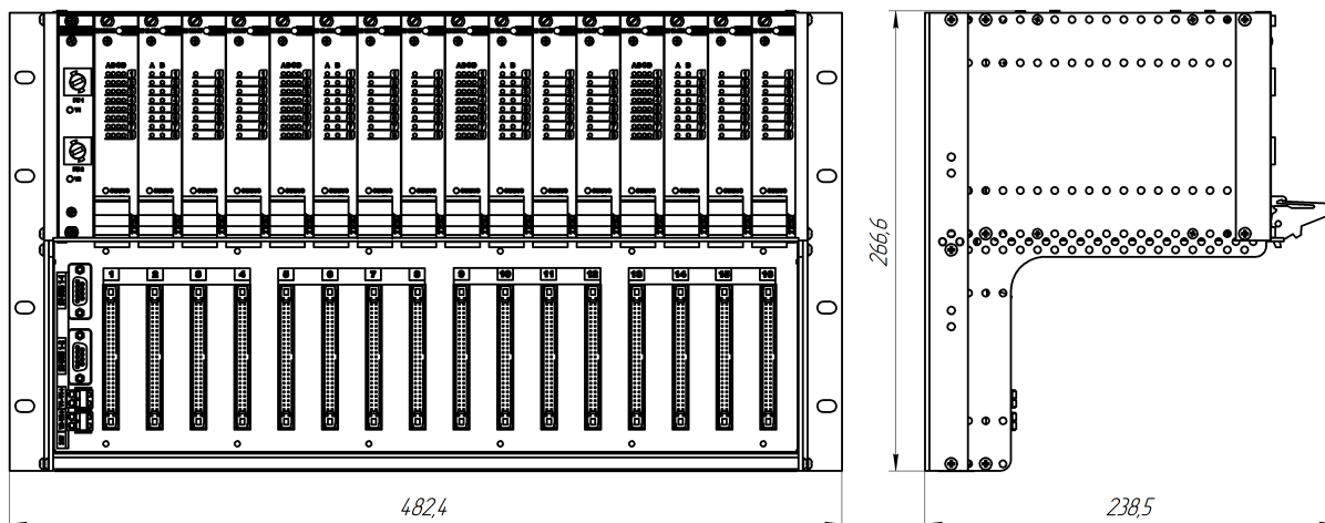
Рисунок 14 – Чертеж общего вида каркаса CR6 IOR с указанием габаритных размеров
