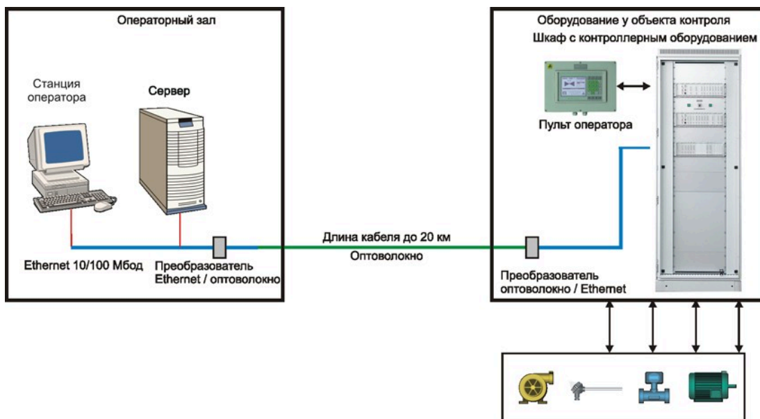
Рисунок 5 – Размещение всего контроллерного оборудования непосредственно с объектом контроля или управления
