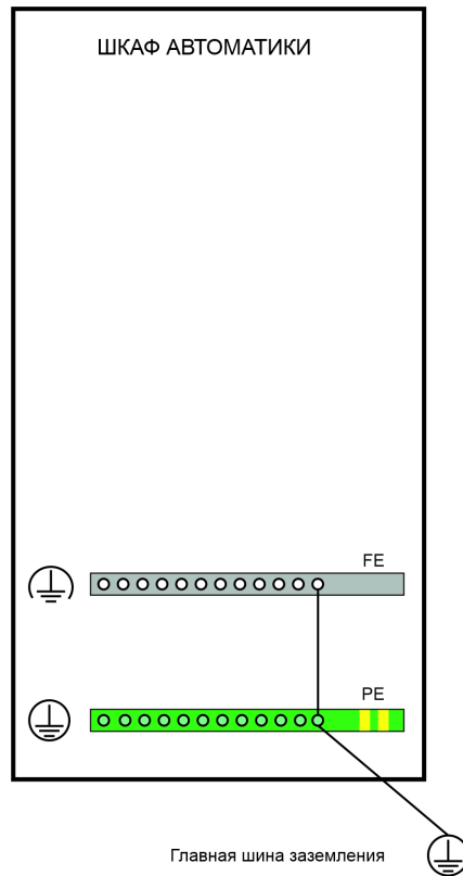
Рисунок 9 – Организация заземления в одном шкафу
