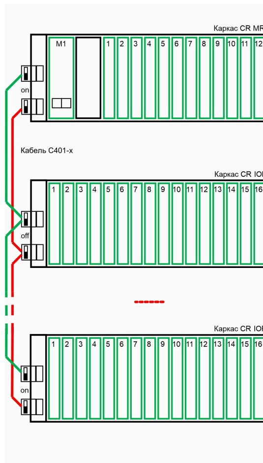
Рисунок 2 – Вариант базовой компоновки контроллера
