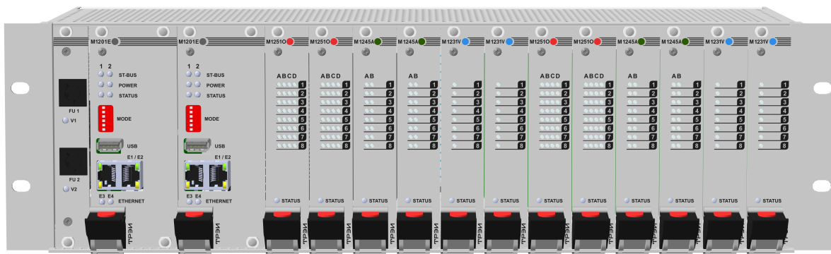
Рисунок 1 – Внешний вид передней панели каркаса CR MR
