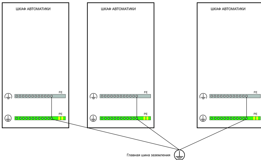
Рисунок 10 – Организация заземления в разных шкафах
