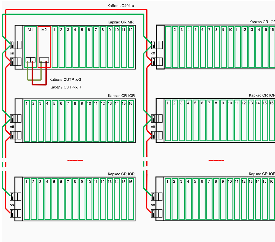
Рисунок 4 – Пример компоновки контроллера с резервированием мастер-модулей
