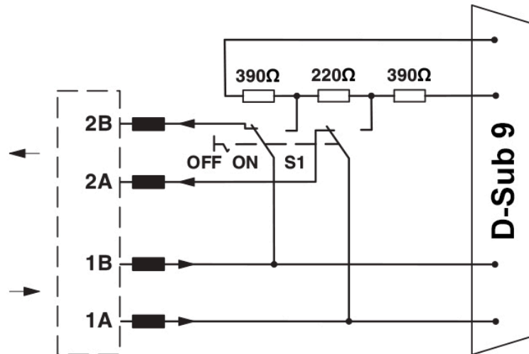
Рисунок 4 – Внутренняя схема соединителя CSB-1
