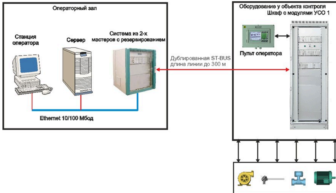
Рисунок 6 – Размещение в помещении операторной только мастер-модулей контроллеров
