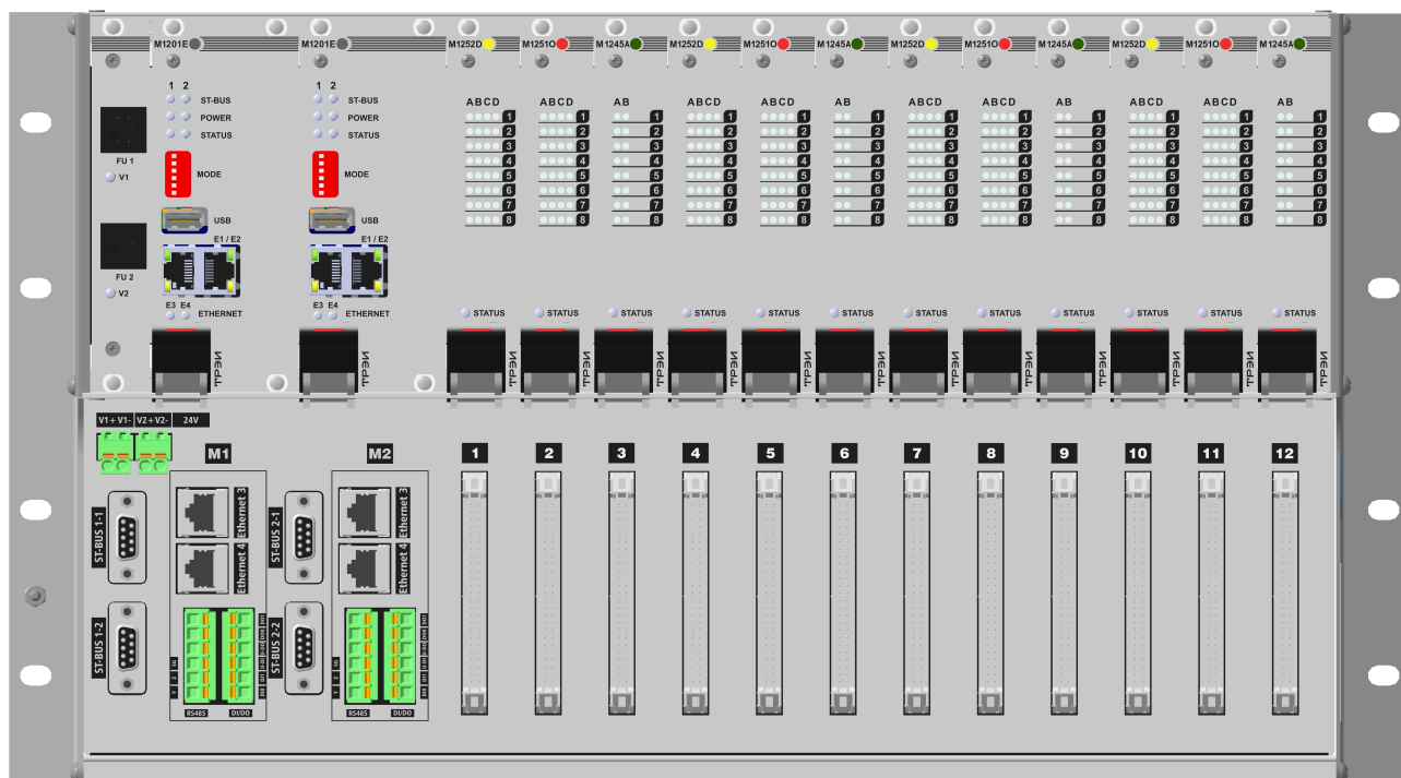
Рисунок 10 – Внешний вид передней панели каркаса CR6 MR
