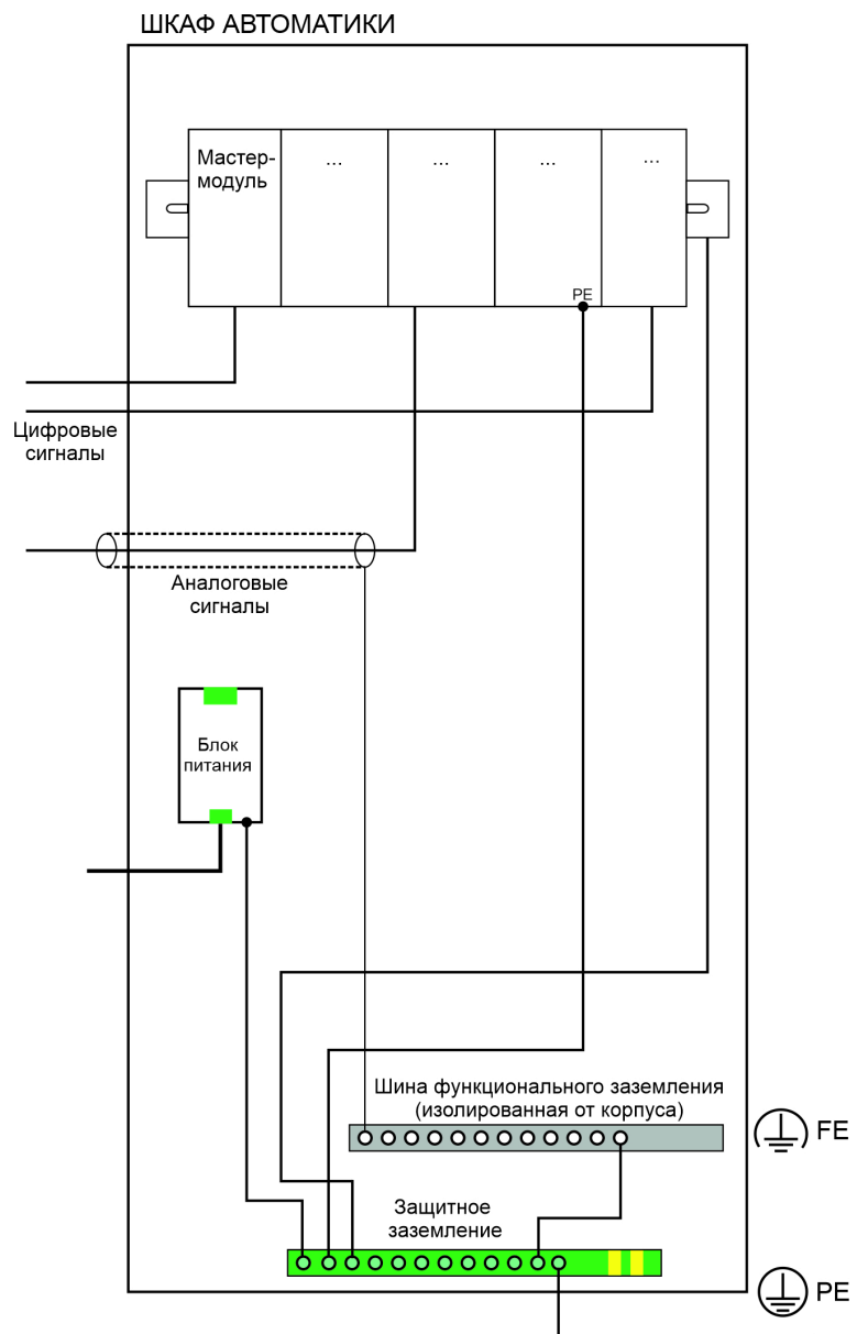
Рисунок 8 – Организация заземления в шкафу
