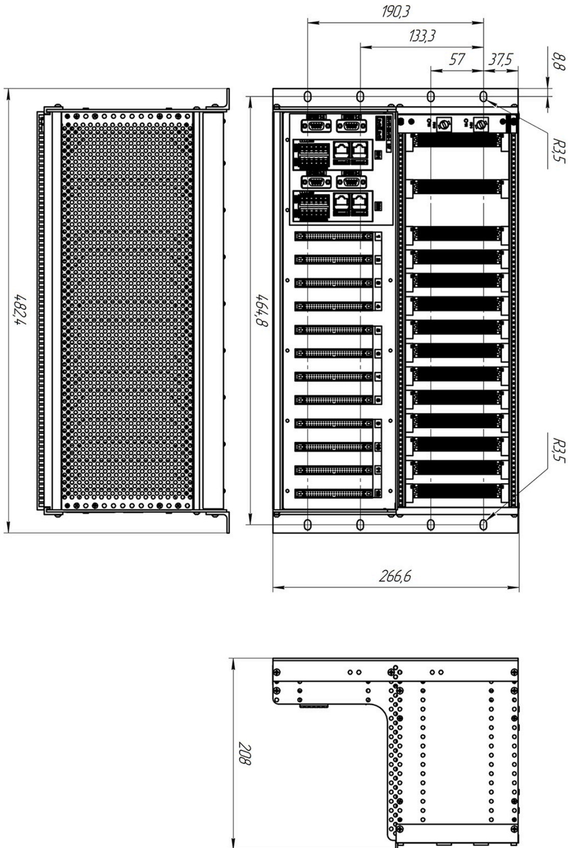
Рисунок 12 – Чертеж общего вида каркаса CR6 MR с указанием габаритных размеров
