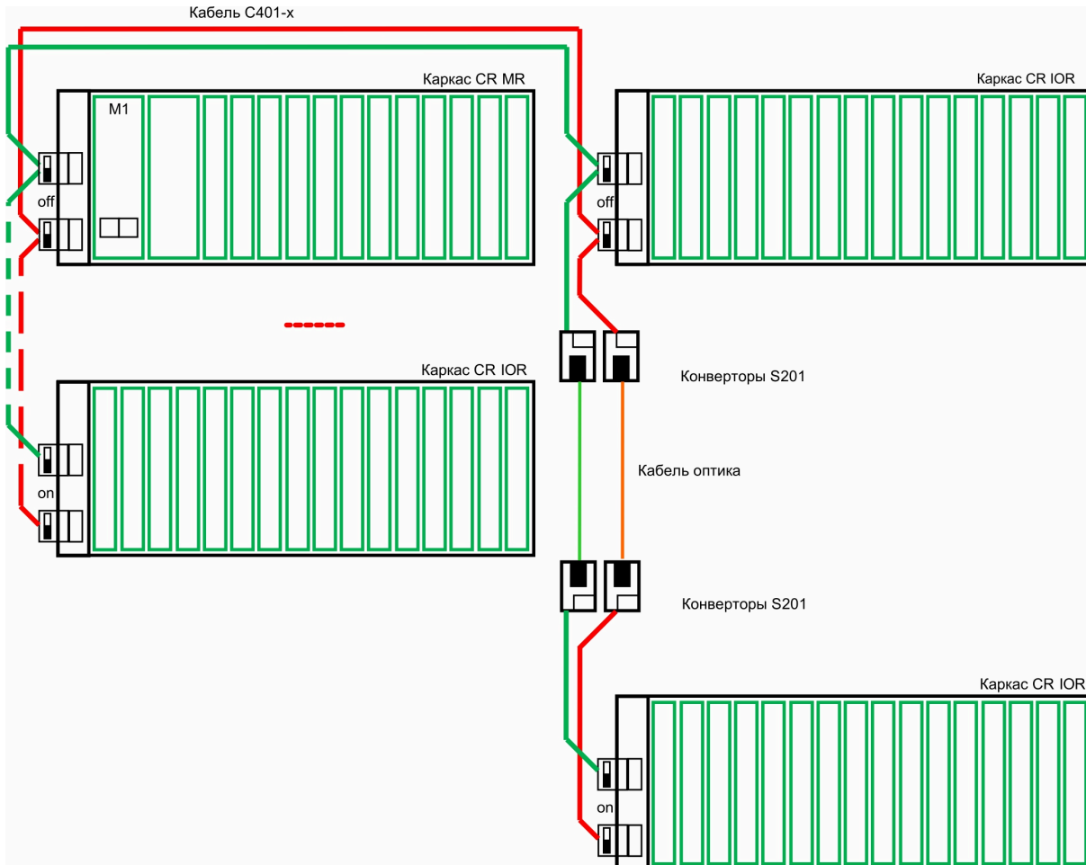
Рисунок 3 – Вариант компоновки контроллера с использованием медиаконвертера S201 при работе по Ethernet
