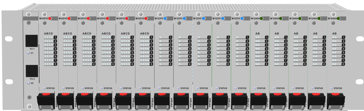
Рисунок 7 – Внешний вид передней панели каркаса CR IOR
